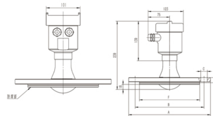
天线3° 结构图
